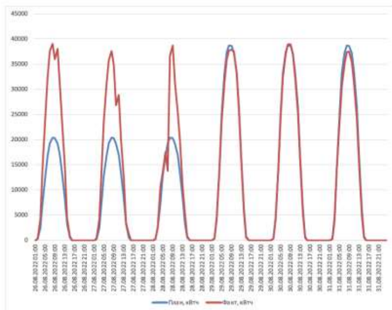
Рисунок 1. График отклонений фактической выработки ЭЭС 50 МВт от плановых значений (26.08.2022–31.08.2022)
