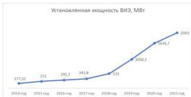
Рисунок 4.1 Динамика установленных мощностей ВИЭ в Республике Казахстан.
