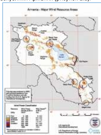
Рисунок 2.1 Карта ветроэнергетических ресурсов Республики Армения
