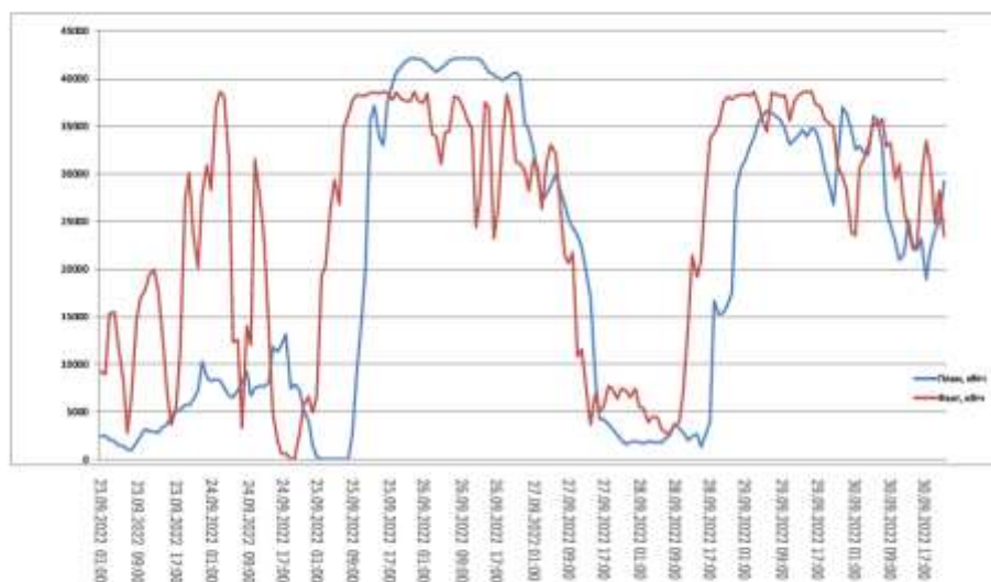
Рисунок 2. График отклонений фактической выработки ЭЭС 48 МВт от плановых значений (23.09.2022–30.09.2022)
