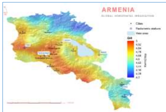
Рисунок 2.2 Карта солнечных ресурсов Республики Армения
